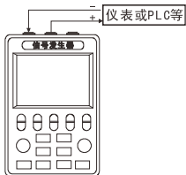
图 2 输出有源电流/电压到仪表或 PLC
