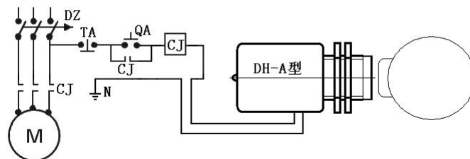
DH-A型用于线包电压AC220V接触器设备保护接线参考图 (适用于容量不大于25A的接触器)
