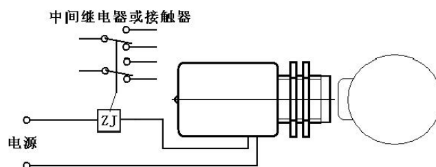
DH系列打滑开关基本接线图
