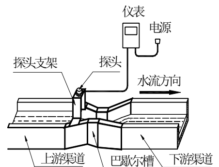
图十二、巴歇尔槽安装在渠道上
