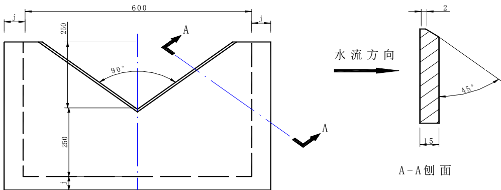
材料：玻璃钢；要求：1，板面光滑、平整、无扭曲；2，三角口缘台要平直、光滑。 j：为测部和底部嵌入渠道测墙的部分，尺寸由安装现场情况确定，一般 5mm。
