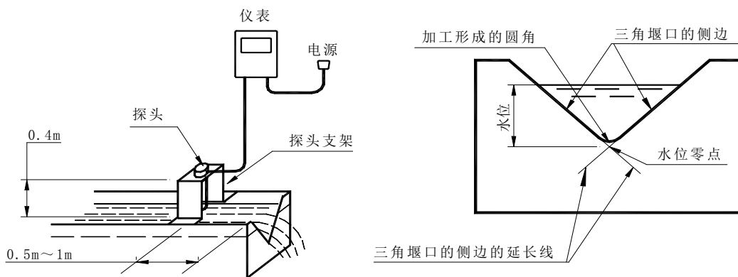
图九、仪表安装在三角堰
